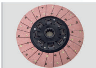
Диск сцепления ведомый 52-1601130 (245 мм) ГАЗ-52, погрузчики, спецтехника Норма упаковки, (шт.) - 5 Вес, (кг.) ..... - 2,65
