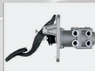
Кран 8648-3514108 ЗИЛ, КАМАЗ, МАЗ тормозной 2-х секционный, подпедальный
