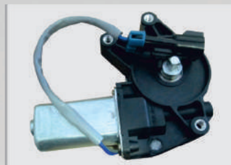
Мотор электростеклоподъемника 1118-6104008 (HW204) 1 , (24В/30Вт) ПРАВЫЙ. ВАЗ 1117-1119, ВАЗ-2123 (Аналог 1118-3730610) Норма упаковки, (шт.) - 20 Вес, (кг.) ..... - 0,55
