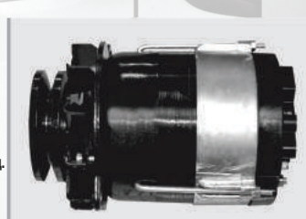
Генератор Г1000В.04.1 (28В/36А) Тракторы: МТЗ-80, 82, Т-70, 70В, 80, 90С, Т-150КС; Дорожно-строительная техника: «Амкор-Ударник», «Арсенал», ТвЭкс, Радицкий машиностроительный завод. Двиг. Д-214, 230, 240, 241, 242, 243, 260 и мод. (аналог: АТ 1000В.04.1) Норма упаковки, (шт.) - 4 Вес, (кг.) ..... - 6,20
