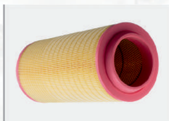
Фильтр воздушный C25710/3 (AM-34-273) JCB JS, JZ КАМАЗ ЕВРО-5 внешний Норма упаковки, (шт.) - 4 Вес, (кг.) ..... - 2,30
