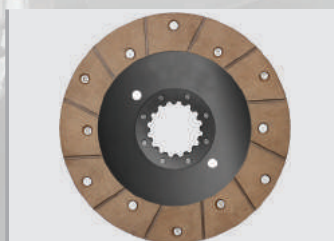
Диск тормозной 80-3502040 (205 мм) КЛЕПАНЫЙ МТЗ-80, 82 Норма упаковки, (шт.) - 20 Вес, (кг.) ..... - 0,66
