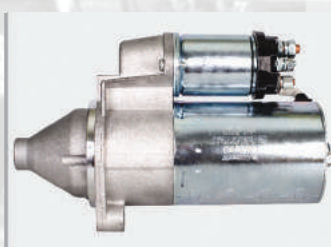
Стартер 5742.3708 (12В/1,7кВт/9 зубьев) ГАЗ-3110 дв. ЗМЗ-406, ГАЗ дв. ЗМЗ 406, -405, УАЗ дв. 409, редукторный (замена 6012.3708) (аналог ЗиТ 5742.3708) Норма упаковки, (шт.) - 4 Вес, (кг.) ..... - 4,20
