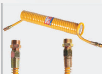
Шланг пневматический (воздушный), 6,5 м; 7,5 м 1868297(8) (M22*1,5) (желтый, красный) ШТУЦЕР M22
