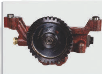
Насос масляный 50-1403010-Б1 Д-243, 245.4, 245.5(С), Д-245.5, 245-16(П), 246.1/4(Евро 3) z=28 Норма упаковки, (шт.) - 6 Вес, (кг.) ..... - 4,67
