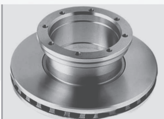
Диск тормозной HD90009348108 (AM-12-027)
