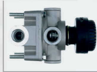
Кран 100-3518010-10 ЗИЛ, КАМАЗ, МАЗ ускорительный с креплением под шумоглушитель Норма упаковки, (шт.) - 20 Вес, (кг.) ..... - 0,82
