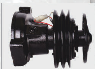
Насос водяной 245-1307015 Д-245.7ЕЗ ГАЗ, ЗИЛ, 12В , «ЕВРО-3» с электромuffтой, 2-х ручьевой Норма упаковки, (шт.) - 2 Вес, (кг.) ..... - 7,70
