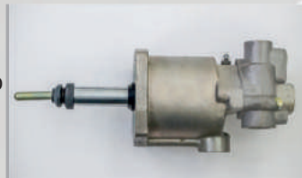
Пневмогидроусилитель 11-1602410-30 МАЗ, МАН, VOLVO аналог WABCO L штока=117мм алюминиевый корпус
