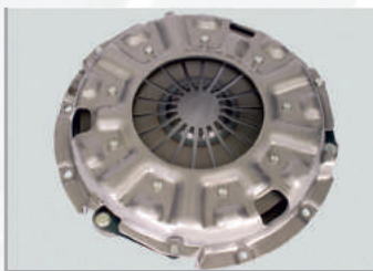
Диск сцепления нажимной (корзина сцепления) 3482001168 (A21R22.1601090) Mf280 ГАЗель-Next КП 330 Нм, дв. Cummins ISF 2.8 (аналог ZF) Норма упаковки, (шт.) - 2 Вес, (кг.) ..... - 9,00
