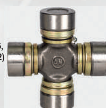
Крестовина карданного вала K-016 (28x72,9) жатки комбайнов Дон-1500, Нива (аналог: НО.51-02.607, 408-2201025, 400-2201025, 52.НО.51-02.607, С29, ВС267-2) в сборе рулевая МАЗ, Урал, КРАЗ, на с/х шарнир 160 Нм Норма упаковки, (шт.) - 80 Вес, (кг.) ..... - 0,45
