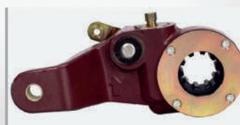
Рычаг регулировочный PT-40-08 ПАЗ-3203, 3204, КАВЗ автомат ПРАВЫЙ, (с установочным комплектом) Норма упаковки, (шт.) - 10 Вес, (кг.) ..... - 3,05
