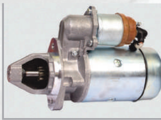
Стартер CT230A1-3708000-10 (12В/1,5кВт) ГАЗ с дв. ЗМЗ-53, ЗМЗ-66, ЗМЗ-66-03, ЗМЗ-71, ЗМЗ-73, ЗМЗ-511, ЗМЗ-513, ЗМЗ-523, ЗМЗ-672, автобусы ПАЗ-672, ПАЗ-3505 Норма упаковки, (шт.) - 2 Вес, (кг.) ..... - 10,00
