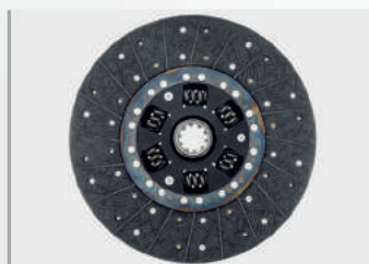
Диск сцепления ведомый 431900-1601130 (AM-28-047) (340мм) ЗИЛ-130, 5301 под лепестковую корзину (340 мм) (аналог: 5301-1601130) Норма упаковки, (шт.) - 5 Вес, (кг.) ..... - 4,60
