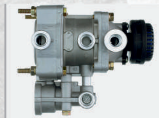
Клапан 25-3522210 КАМАЗ, МАЗ полуприцепа с клапаном обрыва Н/О Норма упаковки, (шт.) - 10 Вес, (кг.) ..... - 1,90
