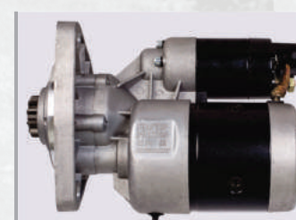
Стартер 925.3708 (12В/0,9кВт) пусковые двигатели ПД-10, 16УД, 350 тракторов: Т-4, 4А, Т-150,-155, -156; ДТ-75, -75М, -75МЛ, -75МП; МТЗ-50Л, -52Л; ТДТ-55, комбайнов «Колос-6», «Сибиряк», КС-6 (Аналог Электром, аналог СТ362А) Норма упаковки, (шт.) - 4 Вес, (кг.) ..... - 3,90
