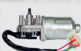
Мотор стеклоочистителя 0 390 243 2011 (HW010A), (12В/40Вт) Газель «Бизнес» (12 В) (Аналог «БОШ») Норма упаковки, (шт.) - 20 Вес, (кг.) ..... - 1,00
