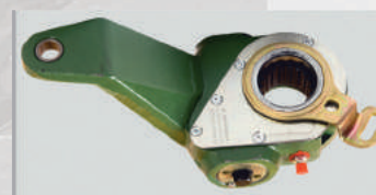
Рычаг регулировочный ZL485D5-3552200 (AM-020-2202017) КАМАЗ, НЕФАЗ ЗАДНИЙ ПРАВЫЙ Норма упаковки, (шт.) - 6 Вес, (кг.) ..... - 3,9
