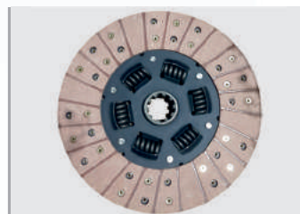
Диск сцепления ведомый 451y-1601130 (451-01-1601130-02) УАЗ дв. 4178, 4218 (под корзину D254 мм, широкий вал 4-хст. КПП) Норма упаковки, (шт.) - 5 Вес, (кг.) ..... - 1,96
