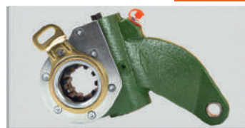
Рычаг регулировочный 80039 КАМАЗ-4326, 43502, 65111, 43118, 63501 ПЕРЕДНИЙ ПРАВЫЙ АВТОМАТ (аналог 9201-3502010-10) 10 зубов Норма упаковки, (шт.) - 6 Вес, (кг.) ..... - 3,45
