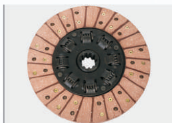
Диск сцепления ведомый 451-1601130 (245 мм) УАЗ-3151, 3741, 3962; УМЗ-421 УАЗ с двиг. УМЗ-4178, 4218 рычажное сцепление Норма упаковки, (шт.) - 5 Вес, (кг.) ..... - 2,10
