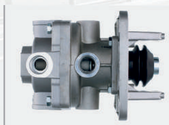
Кран 100-3514108-10 ЗИЛ, КАМАЗ, МАЗ тормозной 2-х секционный подпедальный
