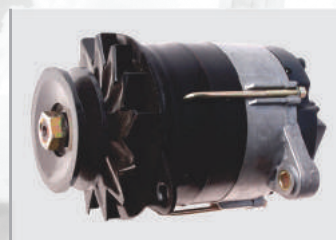
Генератор Г1000В.10.1 (28В/36А) Тракторы: Т-130М, 140, 150К, 170, Т-10 и модификации. Двиг. Д-180, 160, 140 (аналог: АТ 1000В.10.1, 996.3701) Норма упаковки, (шт.) - 4 Вес, (кг.) ..... - 6,10
