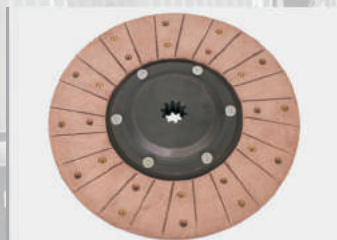
Диск сцепления ведомый T25-1601130-10 (300 мм) Т-40 главной муфты ведомый (10 щлиц) Норма упаковки, (шт.) - 5 Вес, (кг.) ..... - 3,30
