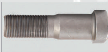
Болт ступицы колеса 54321-3104051 МАЗ М22х1.5х82 короткий ЕВРО (Еврошпилька) Норма упаковки, (шт.) - 10/50 Вес, (кг.) ..... - 0,32
