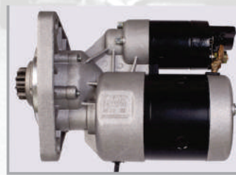
Стартер 9172780 (24В/4кВт) МТЗ-100, МТЗ-102, МТЗ-1025, МТЗ-1005, МТЗ-1221, МТЗ-1522, Т-150КС, Зил-5301 (Бычок), ПАЗ, ГАЗ-33081 «Садко», ГАЗ-3309, ГАЗ-33104 «Валдай», виброкоток ВГ-1201, МАЗ-4370, Амкордор., дв: Д-245, Д-260Е2, Д-245Е2 (Аналог Magnetop) Норма упаковки, (шт.) - 4 Вес, (кг.) ..... - 5,70
