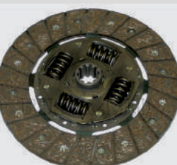
Диск сцепления ведомый AM.409-1601130 (AM-28-055)
