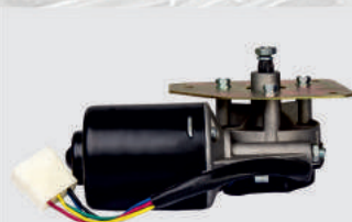
Мотор стеклоочистителя 13.52305100-02 (HW004B), (24В/50Вт) КамАЗ, БелАЗ Норма упаковки, (шт.) - 10 Вес, (кг.) ..... - 1,82
