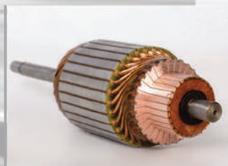
Якорь стартера СТ230-3708200
