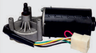
Мотор стеклоочистителя 16.3730 (HW004) (24В/20Вт) ГАЗ, ЗИЛ, КамАЗ, МАЗ, КрАЗ, БелАЗ, Моаз Норма упаковки, (шт.) - 15 Вес, (кг.) ..... - 1,71
