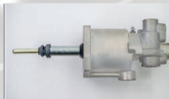
Пневмогидроусилитель 11.1602410-10 УРАЛ дв. ЯМЗ под лепестковое сцепление (181, 182, 183, 184) алюминиевый корпус (аналог 11.1602410-10, 11.1602410-10P, 11.1602410-11)
