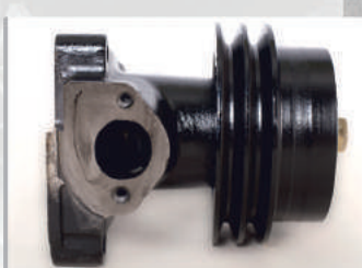
Насос водяной 245-1307010-А1-07 ГАЗ-3310 «Валдай» ММЗ Д-245.7Е2 «Евро-2» Норма упаковки, (шт.) - 2 Вес, (кг.) ..... - 7,65
