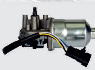
Мотор стеклоочистителя 3163-5205100 (HW010), (12В/40Вт) УАЗ-3163 Норма упаковки, (шт.) - 20 Вес, (кг.) ..... - 1,06
