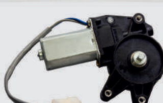
Мотор электростеклоподъемника 2110-3730610 (HW202), (24В/30Вт) ПРАВЫЙ ВАЗ 2108-2115 Норма упаковки, (шт.) - 20 Вес, (кг.) ..... - 0,55
