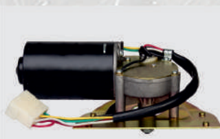
Мотор стеклоочистителя 272.5205.100 (HW006), (24В/50Вт) КамАЗ «Евро» Норма упаковки, (шт.) - 10 Вес, (кг.) ..... - 2,10
