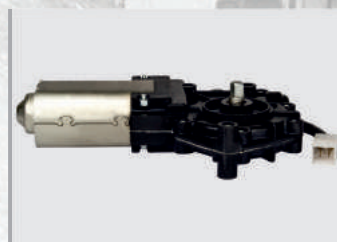
Мотор электростеклоподъемника 20.3780-01 (HW212) 1 , (24В/8Вт) ПРАВЫЙ. ВАЗ-2109, 2110 (Аналог 2110-3730610) Норма упаковки, (шт.) - 20 Вес, (кг.) ..... - 0,90
