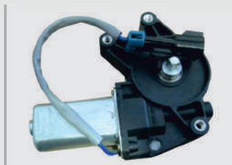
Мотор электростеклоподъемника 1118-6104009 (HW203) 1 , (24В/30Вт) ЛЕВЫЙ. ВАЗ 1117-1119, ВАЗ-2123 (Аналог 1118-3730611) Норма упаковки, (шт.) - 20 Вес, (кг.) ..... - 0,55
