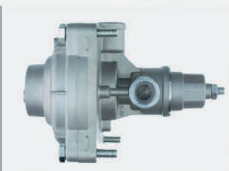
Клапан 100-3522110 ЗИЛ, КАМАЗ, МАЗ, КРАЗ однопроводный управления тормозами прицепа Норма упаковки, (шт.) - 10 Вес, (кг.) ..... - 2,00
